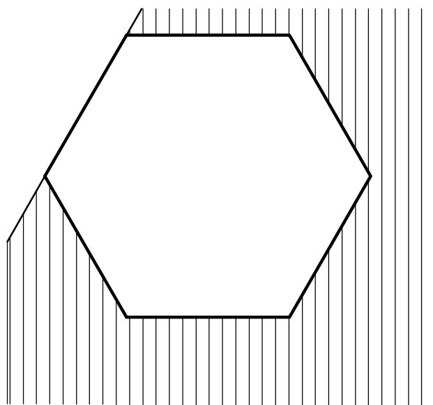
POLÍGONO CÓNCAVO
